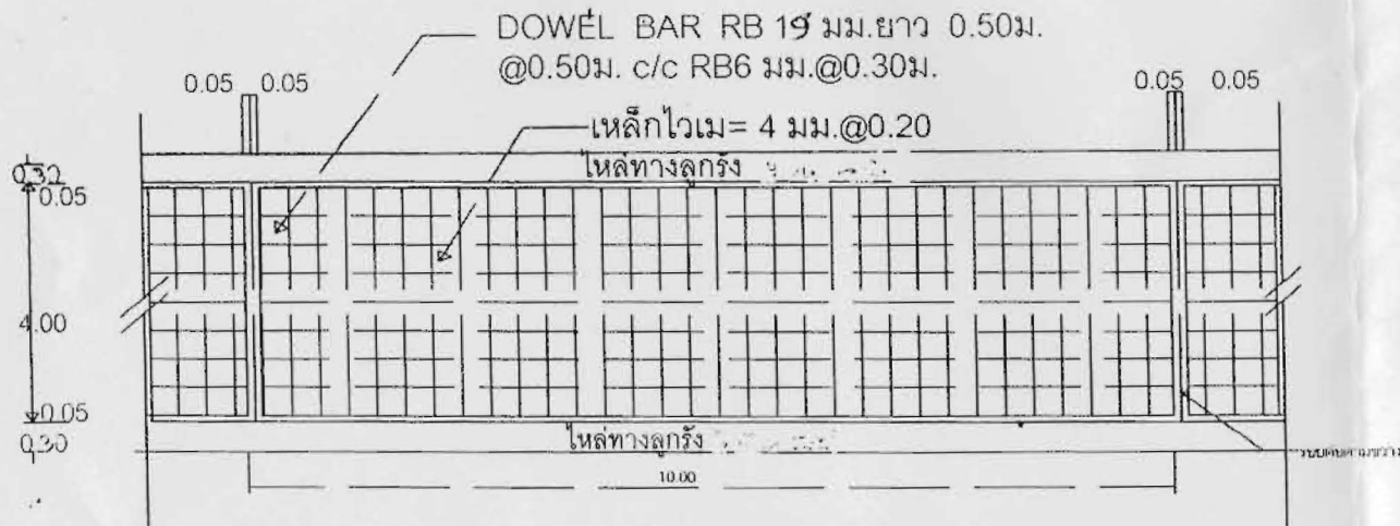
รูปแปลนผิวจราจรคอนกรีต
